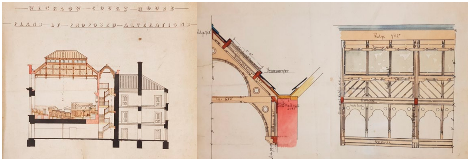
Líníocht ailtire de theach cúirte Chill Mhantáin (1876). Cartlann Contae Chill Mhantáin:
